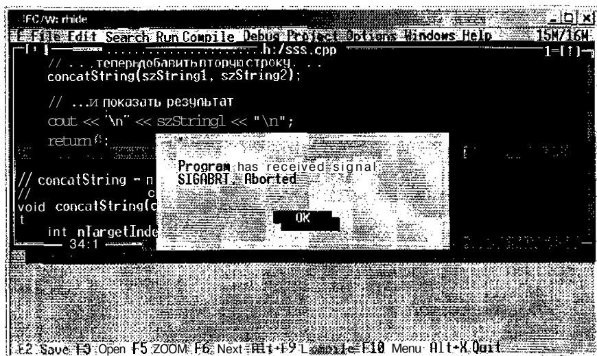
Рис. 11.4. Ошибка в функции concatstring() заставляет программу аварийно завершаться
