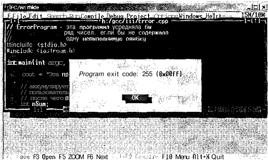
Рис- 11.2. Код выхода 0xff означает, что программа завершилась аварийно
