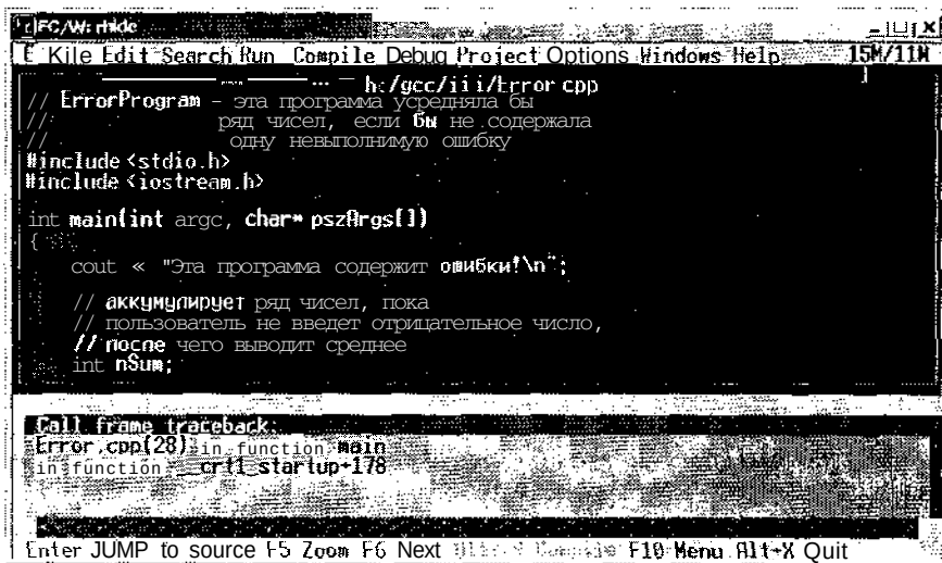
Рис. 11.3. Редактор rhide способен вычислить, в какой части программы возникла ошибка
